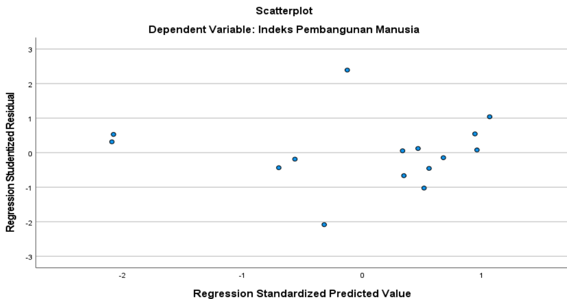
Gambar 6. Uji Heteroskedastisitas
